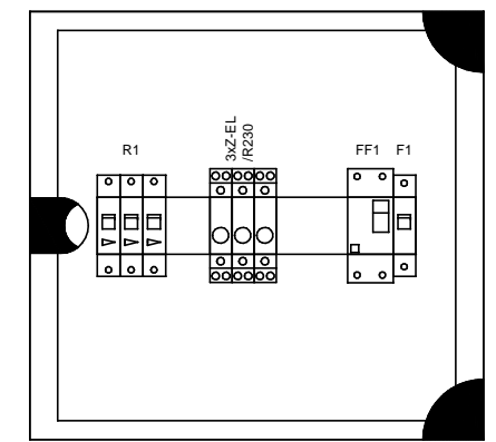
KLV-U-1/14-D - szafka podtynkowa z drzwiami plastikowymi białymi na 14 modułów, zamykana na kluczyk
