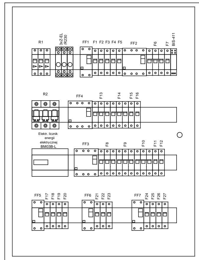
BF-U-3/96-P - rozdzielnica podtynkowa z drzwiami metalowymi na 96 modułów, zamykana na kluczyk
