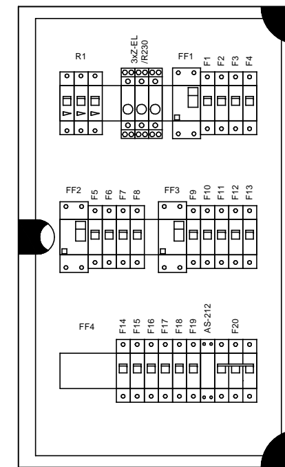
KLV-U-3/42-D - szafka podtynkowa z drzwiami plastikowymi białymi na 42 moduły, zamykana na kluczyk
