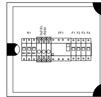
KLV-U-1/14-D - szafka podtynkowa z drzwiami plastikowymi białymi na 14 modułów, zamykana na kluczyk
