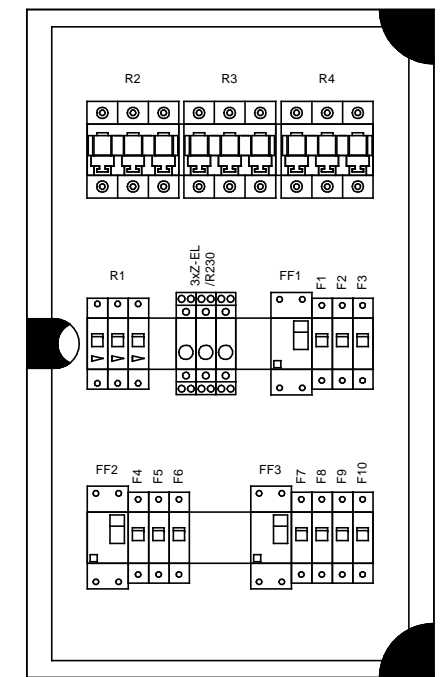
KLV-U-3/42-D - szafka podtynkowa z drzwiami plastikowymi białymi na 42 moduły, zamykana na kluczyk
