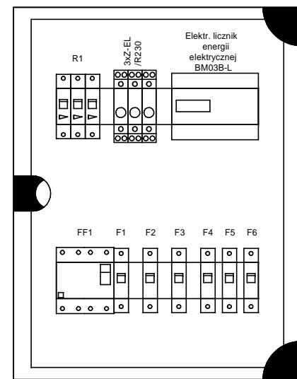
KLV-U-2/28-D - szafka podtynkowa z drzwiami plastikowymi białymi na 28 modułów, zamykana na kluczyk
